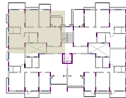
KEY PLAN TYP 1 ST & 3 RD FLOOR
